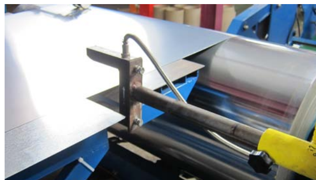
Инфракрасный Сенсор DS-100 применяется на Машинах для Отделки Стального Полотна
